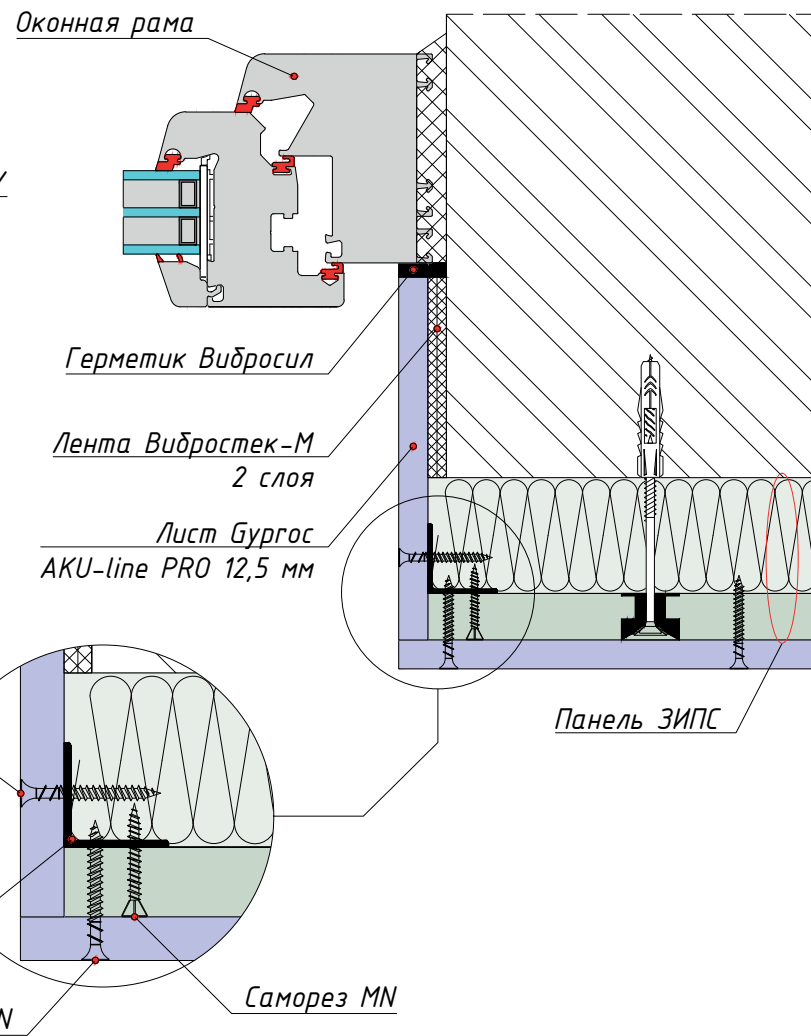
Узел 2.9 Оформление вертикального оконного откоса
