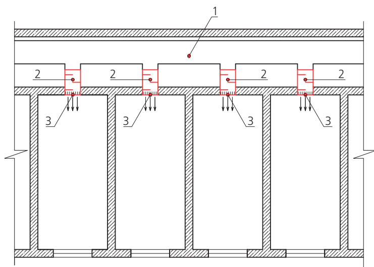
Рис. 1. Фрагмент плана гостиной после установки шумоглушителей: 1 – вентиляционный канал; 2 – шумоглушитель ГПП 500×500/1000; 3 – концевые воздухораспределительные устройства
