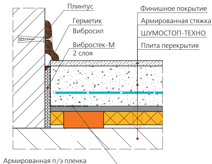
Рис. 2. Звукоизоляция пола с применением панелей ШУМОСТОП-ТЕХНО под стяжкой
